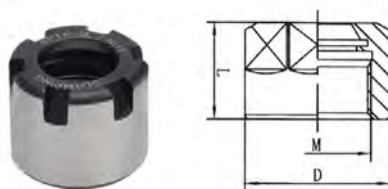
ER-M 型螺帽 ER-M Nuts
