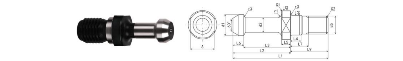
SR 拉钉 SR Pull Stud
