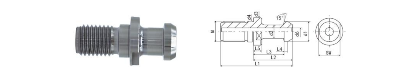
日本 JIS B6339 拉钉 Japan JIS B6399 Pull Stud
