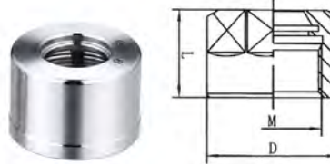
ER-GSK 型螺帽 ER-GSK Nuts
