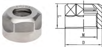
ER-A 型螺帽 ER-A Nuts
