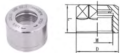
ER-GER 型螺帽 ER-GER Nuts
