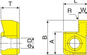
图A 单头 Fig. A Single-head
